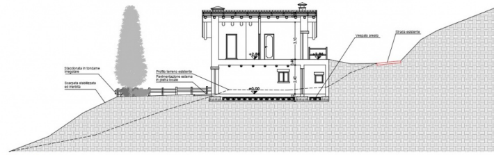
SEZIONE B-B
